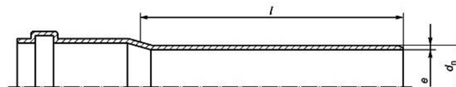
Рисунок 2. Эффективная длина труб
